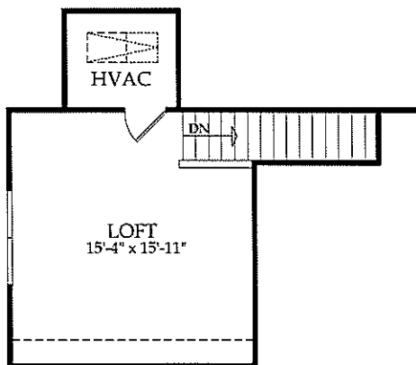
Loft Option
