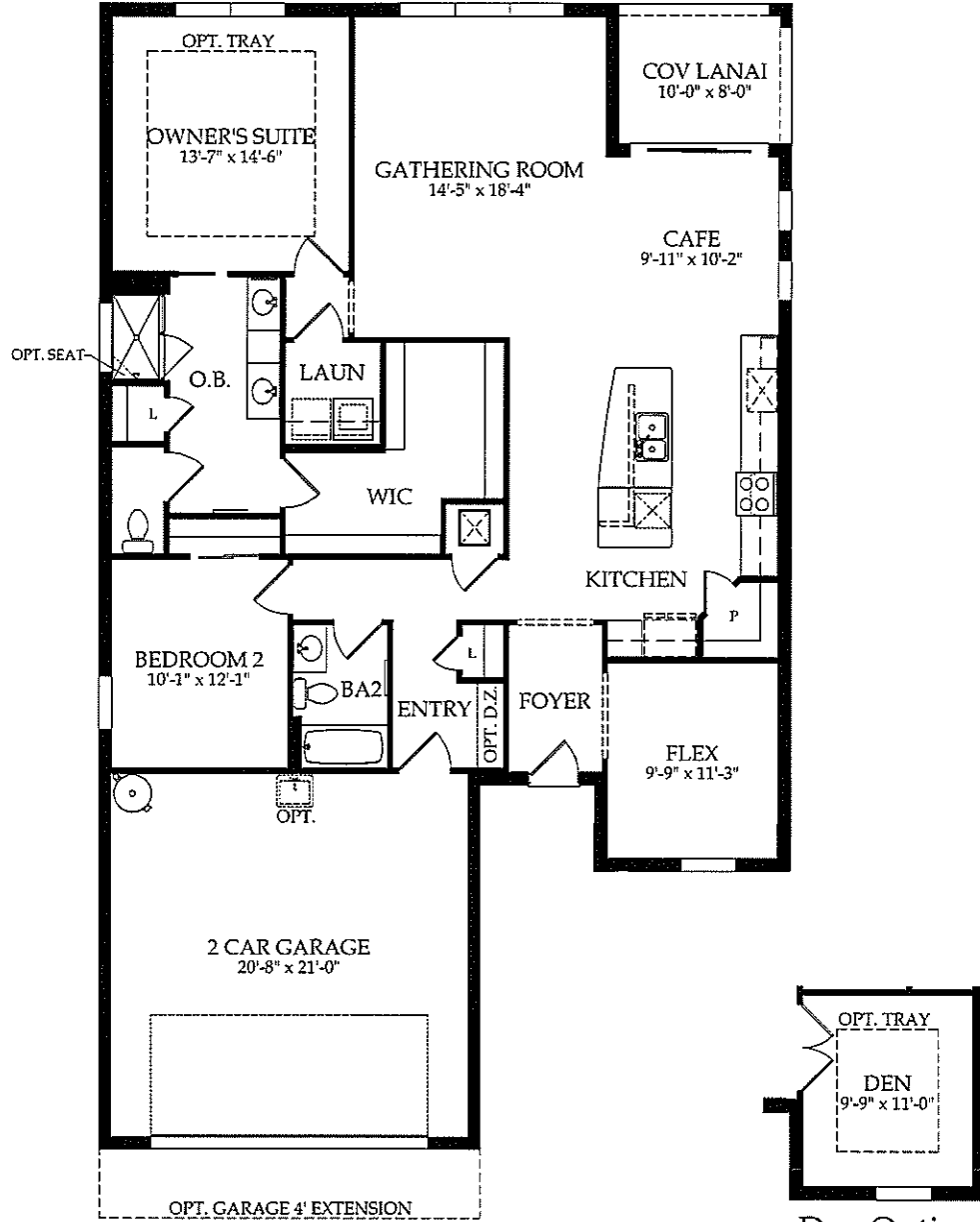
Den Option
