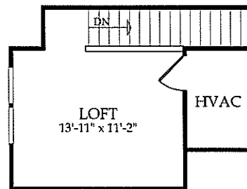
Loft Option
