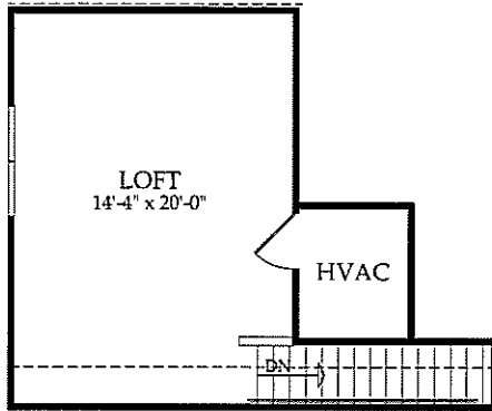
Loft Option
