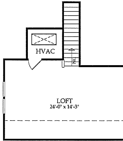
Loft Option
